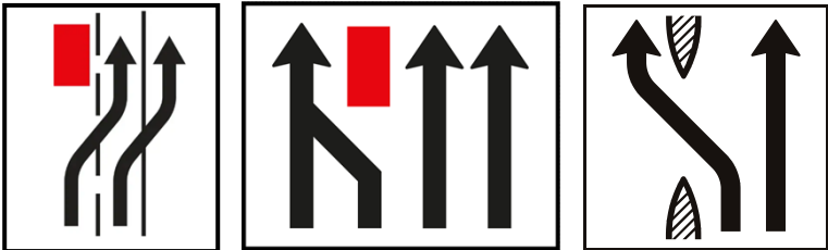
4.77.3 Disposition du tracé des voies de circulation aux abords d'un chantier (exemples) (art. 59)
