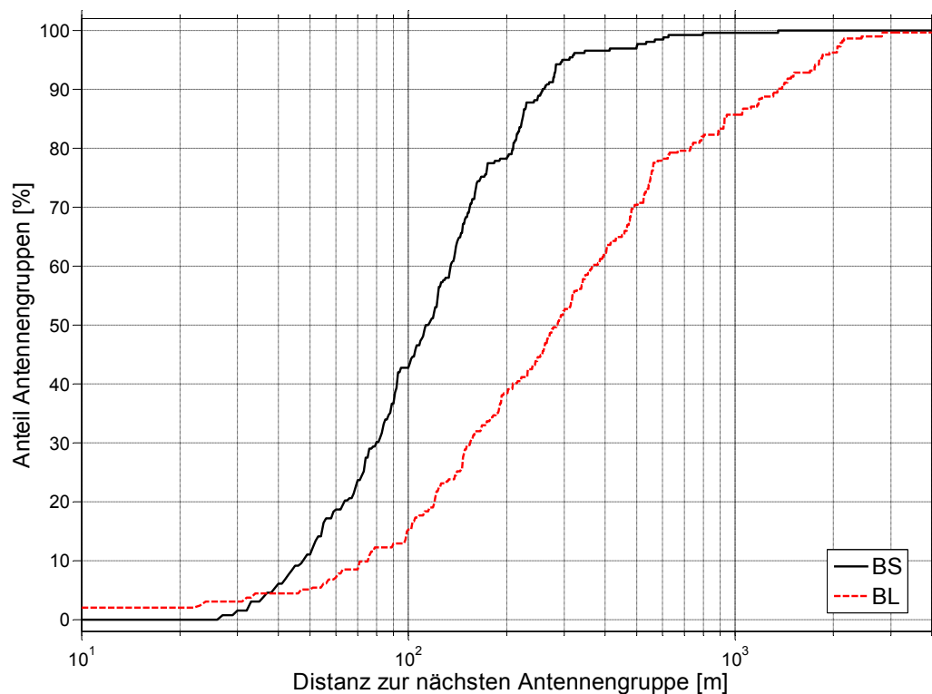
Abbildung 1: Horizontaler Abstand zur nächsten Antennengruppe 8 (Summenhäufigkeitsverteilung)
