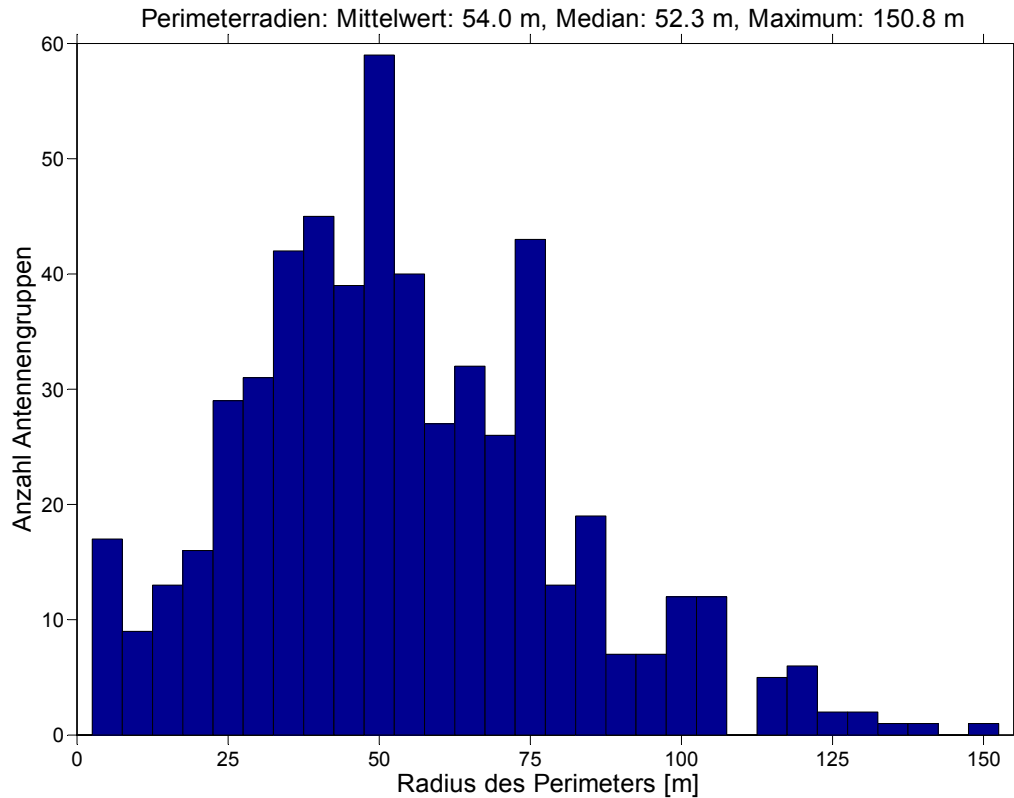
Abbildung 2: Perimeterradien
