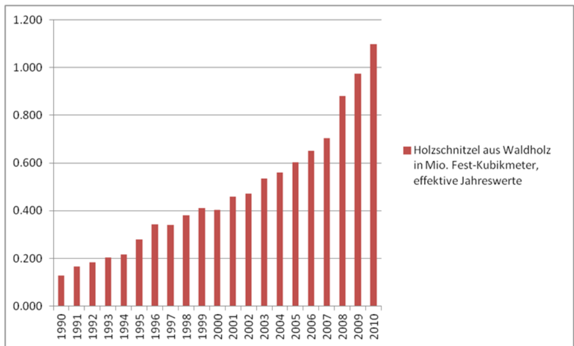
Abbildung 1: Holzsnitzel aus Waldholz in Mio. m 3 – Quelle: Auswertung zur Holzenergiestatistik 2010 [Basler & Hofmann 2011]
